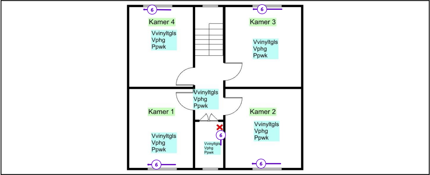
Legende van plan 1.9: locatie te onderzoeken radiatoren +1
